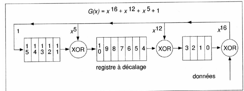
Circuits permettant de calculer R(x)
