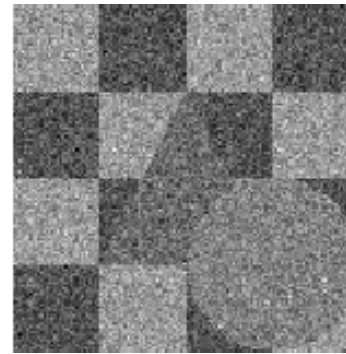
Image bruitée
