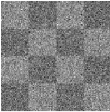
Image bruitée
