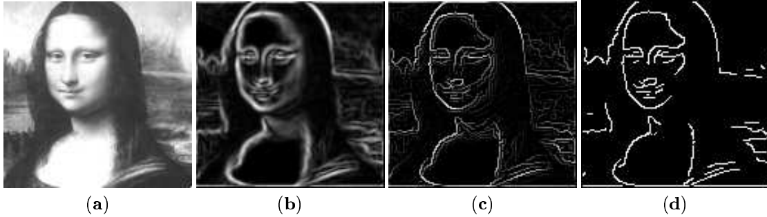
FIG. 2 – (a) Image originale mona.pgm . (b) Rehaussement de Canny (avec un filtre Gaussien d'écart type \sigma = 1 ). (c) Résultat de la suppression des non maximums (étape 2). (d) Résultat du seuillage par hystérésis avec \tau_l = 70 et \tau_h = 90 (étape 3).
